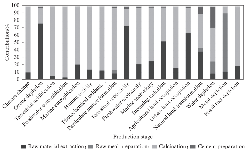
图4 水泥生产各阶段对环境的影响类别的贡献
