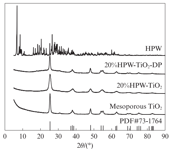
图1 HPW及3种催化剂样品的XRD图谱
