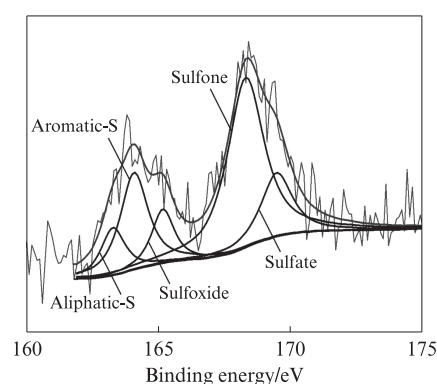
(d) S2p spectral lines of MSS with 20%HPW-TiO 2
