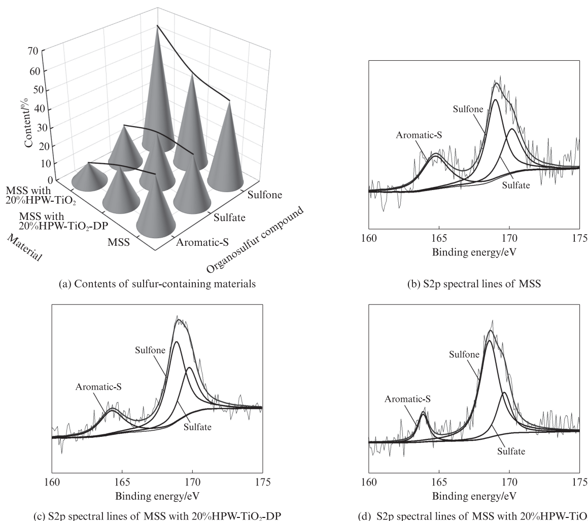
图7 煅烧 320 °C 后掺/未掺介孔 HPW-TiO 2 催化剂的 MSS 中含硫物的含量及 S2p 谱线
