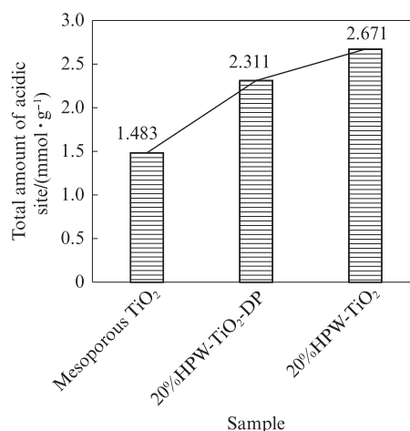
图 4 介孔 TiO 2 、20%HPW-TiO 2 和 20%HPW-TiO 2 -DP 样品的酸性位点总量
