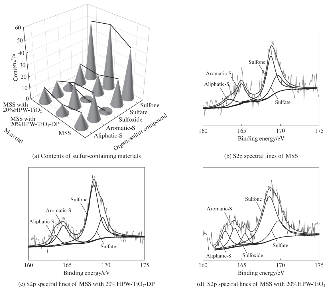
图6 煅烧260℃后掺/未掺介孔HPW-TiO 2 催化剂的MSS中含硫物的含量及S2p谱线
